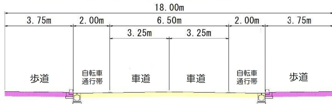
標準断面図
